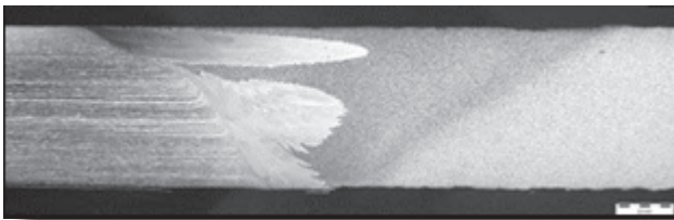
Figura 9. Sección metalográfica de una soldadura realizada entre acero al carbono S355 de 8 mm. de espesor y acero inoxidable dúplex S32205.
