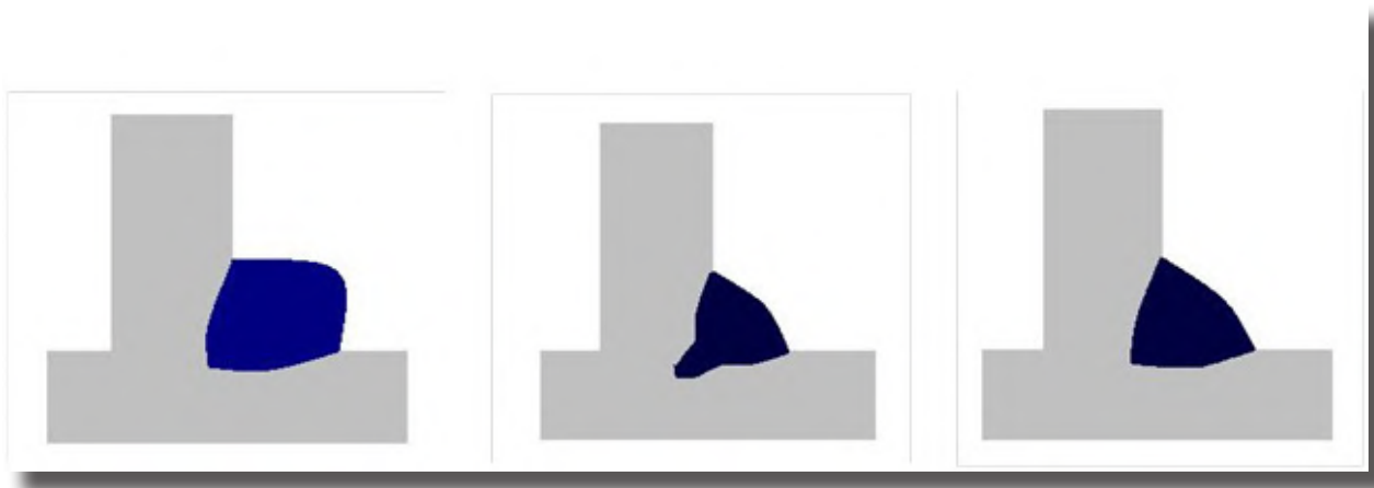
Figura: efecto del CO 2 , el argón y las mezclas de Ar/CO 2 en el perfil de penetración para soldadura MAG.
