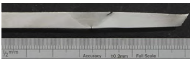
Figura 7. Una sección metalográfica a través de un FSW intencionalmente defectuoso en acero DH36 de 6 mm. de espesor. La zona del fallo está en el metal principal al lado derecho de la muestra.
