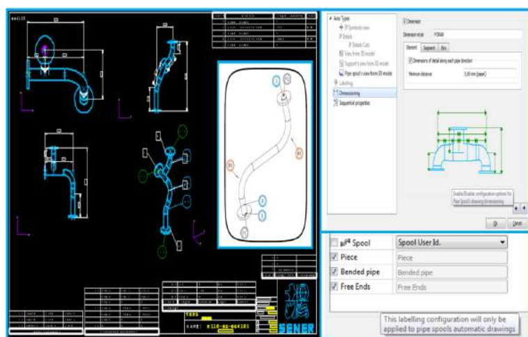
Figura 4: La nueva zona en la plantilla de planos permite configurar las dimensiones necesarias en esa área del plano automático.
