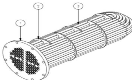
Figura 7.- Haz tubular en U con disposición triangular mostrando 1-placa; 2-deflector o baffle; 3-haz tubular.
