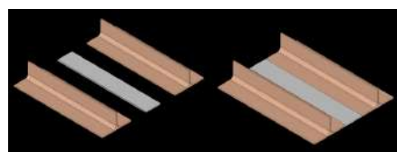
Figura 10 (arriba) Esquema de los canales laminados y las placas espaciadoras. (Abajo) Ejemplo de un Panel Reforzado Integralmente totalmente forjado.
